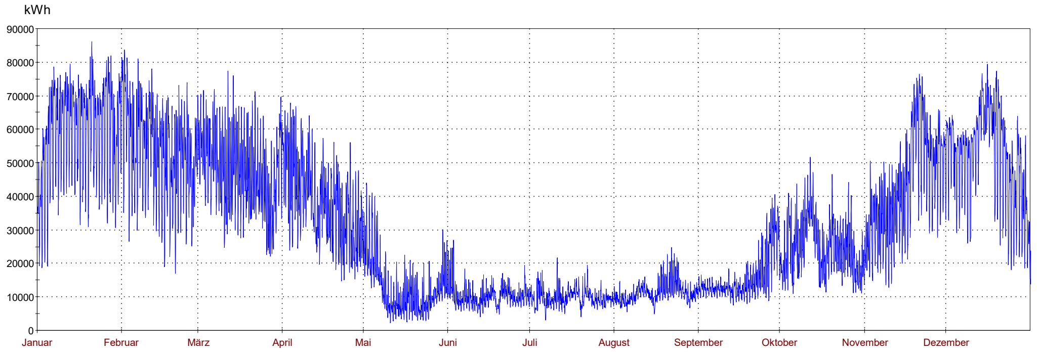
Jahreshöchstlast 86.132 kW - Lastverlauf als stündliche Leistungsmessung (Maximum am 21.01.2022 07:00 Uhr)
