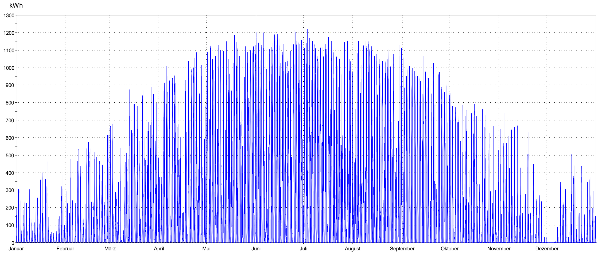
Summe aller Einspeisungen in die Niederspannungseben 5.784.014 kWh mit zeitlichem Verlauf
