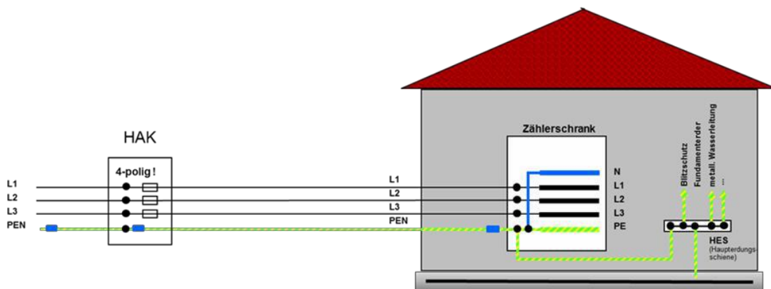
Abb. 16: Anschlussvariante bei SWE zur Außenanschlusstechnik (beispielhafte Darstellung)
